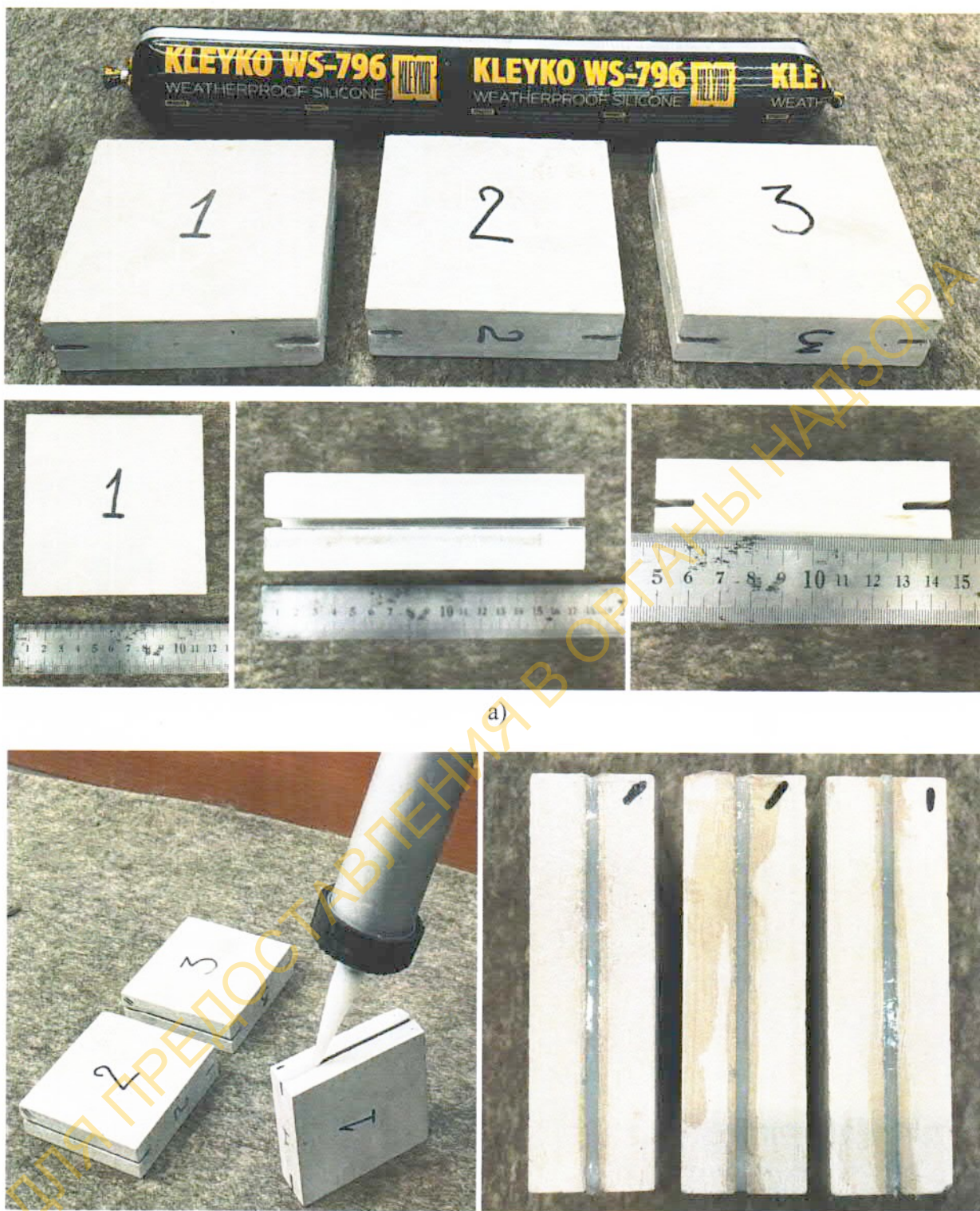
Рисунок 1. Образцы из плитки из натурального камня Гохара: а) до внесения герметика в пазы плитки; б) после внесения герметика в пазы плитки
